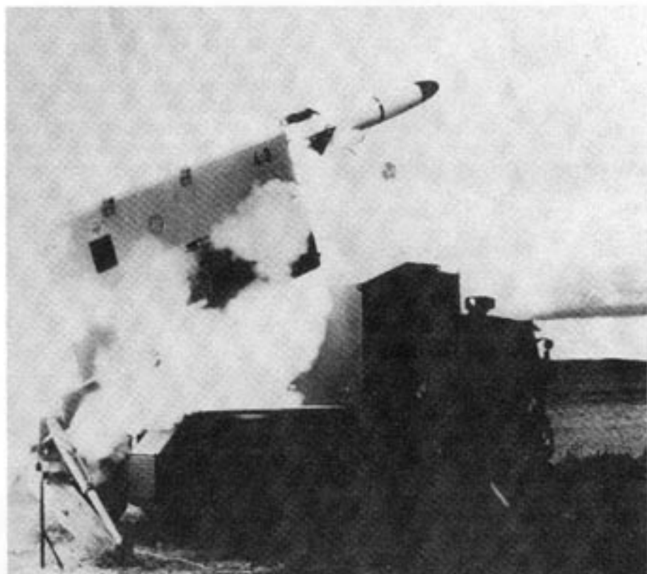
Sveriges motsvarighet till den välkända franska Exocet-roboten är RBS15. Här testas en RBS15 från en mobil plattform. För trettio år sedan träffade en robot nästan aldrig ett mål, idag träffar de alla flesta robotarna målet, på grund av den nya elektroniken.
